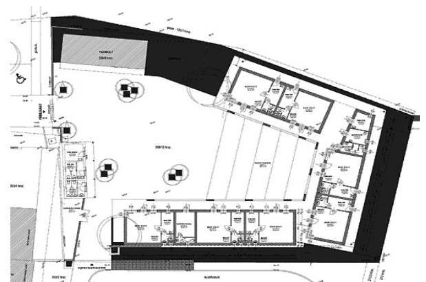
A piactér és az üzletsorok alaprajza
